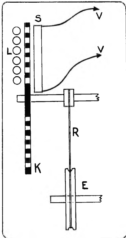
L = Lampgroep. S = Seleniumcel V = Toevoerdra- den naar versterkers en luidsprekers K = Klankschijf. R = Riemaandrijving. E = door electromotor aangedreven as
